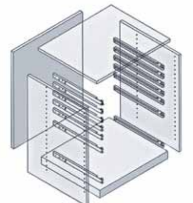
Cassetto con guide da avvitare Drawer with runners to be screwed Tiroir avec coulisses à visser Schublade mit Führungsschienen Cajon con guías a atornillar
